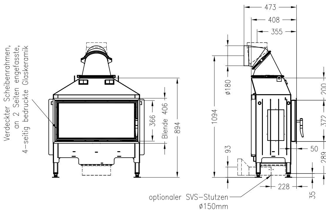
Vorderansicht M ~1:20
